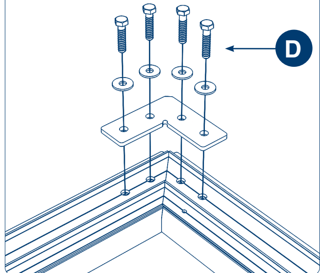
Рис. 11.1. Вид 1
