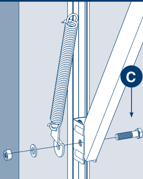
Рис. 8.2. Вид 2
