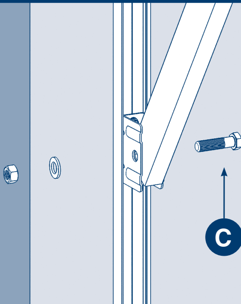
Рис. 8.1. Вид 1
