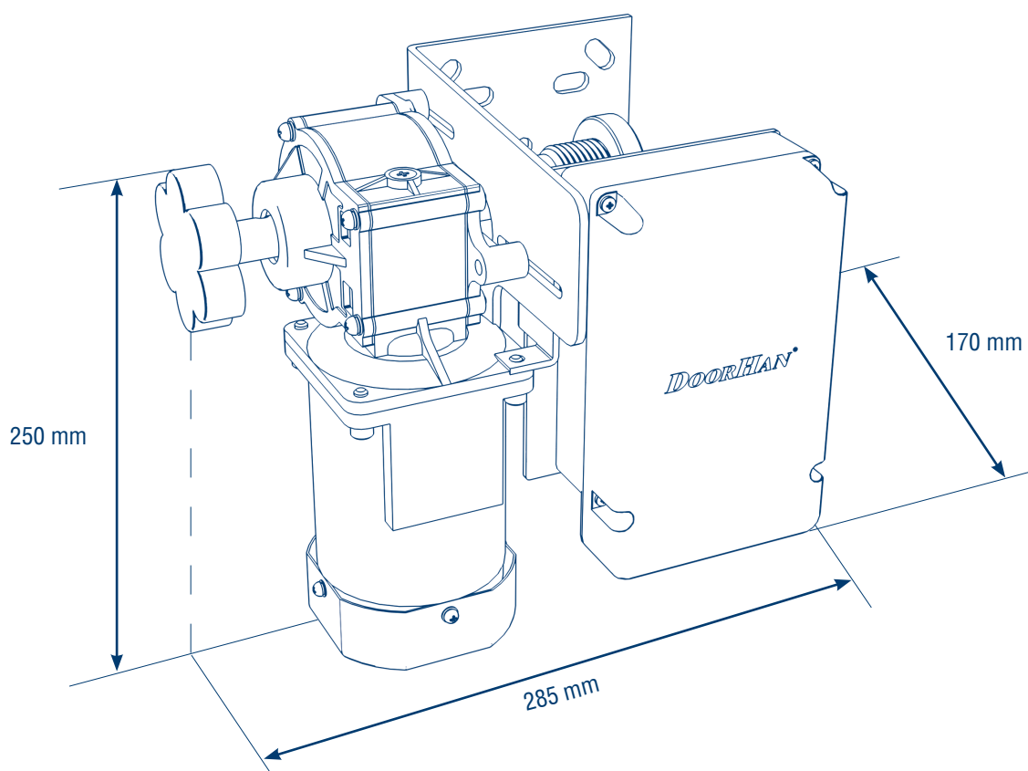
Рис. 1.2. Габаритные размеры / Fig. 1.2. Overall dimensions
