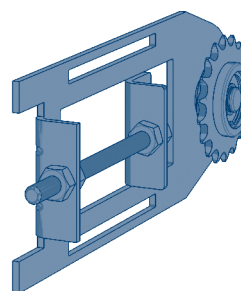
Рис. 6.2.2. Пластина натяжителя цепи
