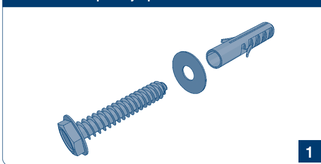
Рис. 6.1.18. Саморез-глухарь 8 × 70 мм
