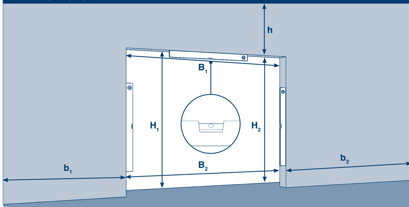
Рис. 8.1.1. Параметры проема
