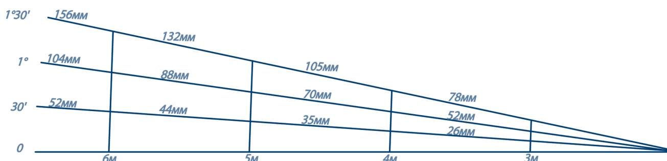
Рис. 7.2.5. Угол наклона направляющей балки
