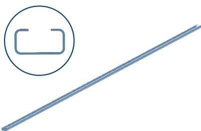
Рис. 6.5.1. С-профиль
