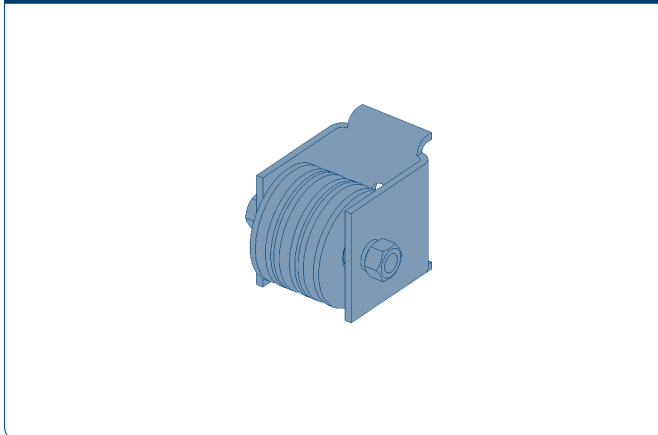
Рис. 6.4.3. Ролик противовеса в сборе
