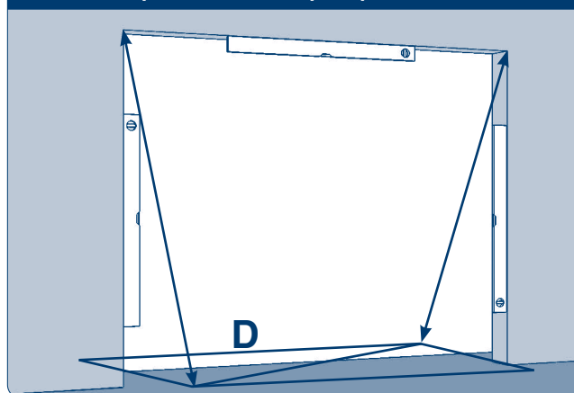
Рис. 7.1.4. Вертикальность сторон проема
