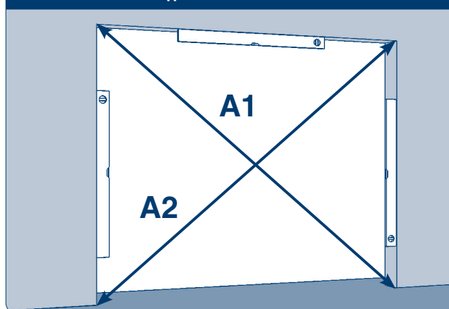
Рис. 7.1.2. Разность диагоналей
