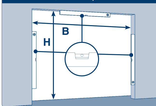
Рис. 7.1.1. Световой/монтажный проем
