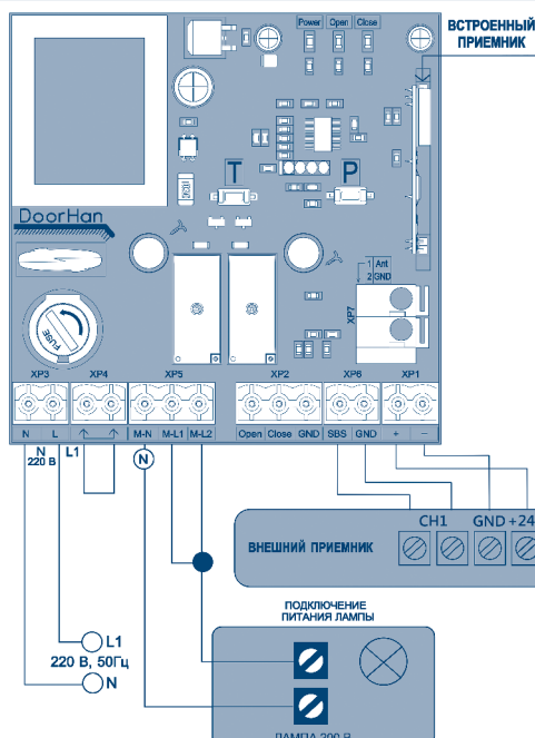
Рис. 2. Схема подключения освещения и внешнего радиуправления
