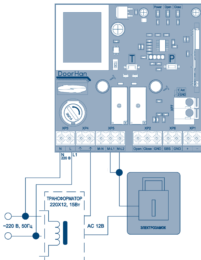
Рис. 3. Схема подключения электрозамка
