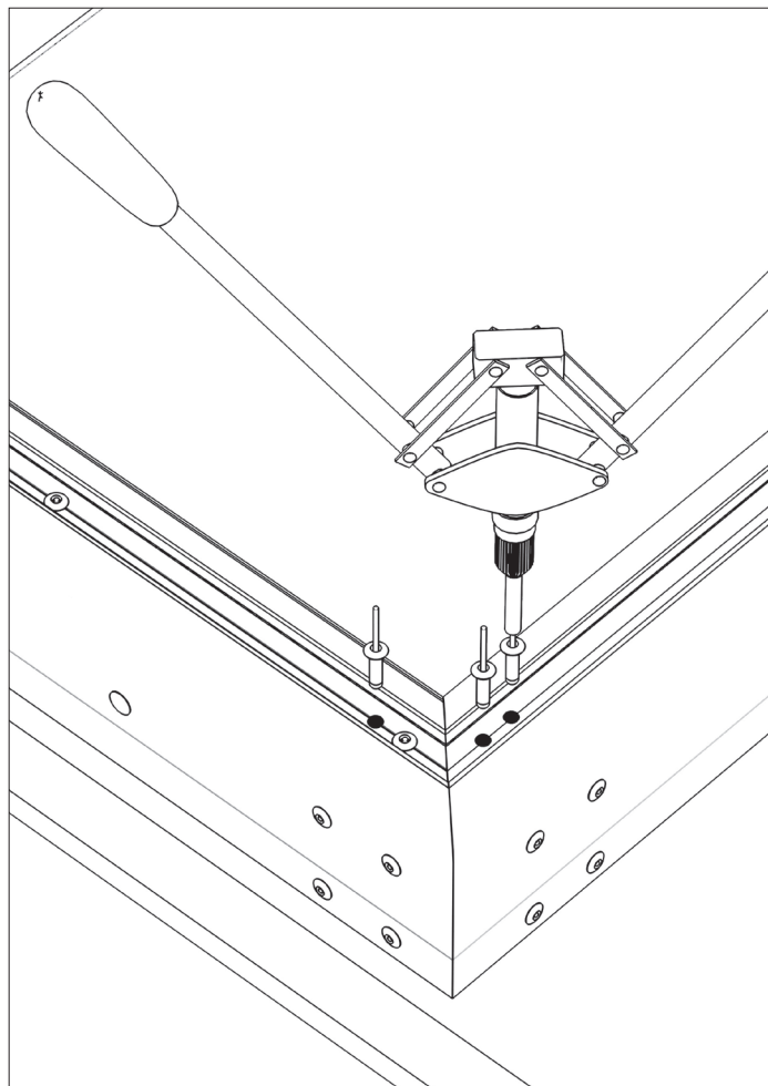
7.2. В просверленные отверстия \varnothing 4,2 мм установите заклепки \varnothing 4 мм.
