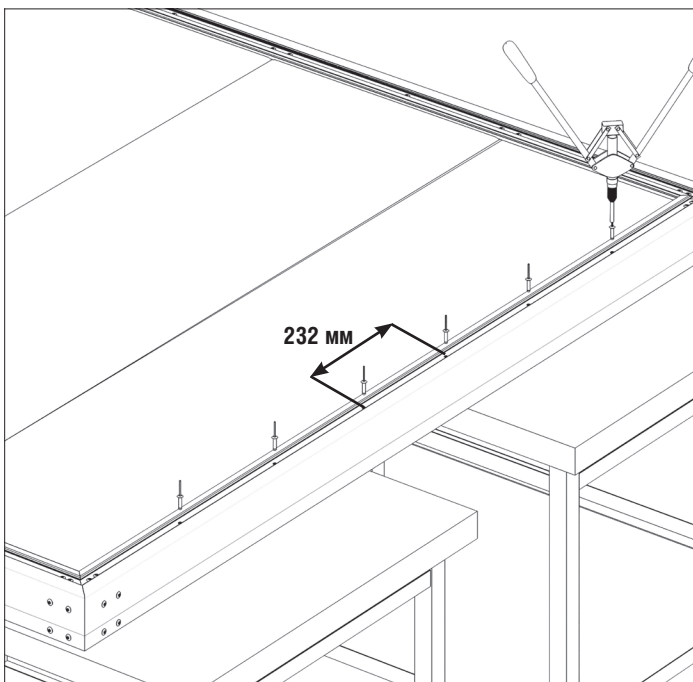
9. В просверленные отверстия \varnothing 4,2 мм установите заклепки \varnothing 4 мм.
