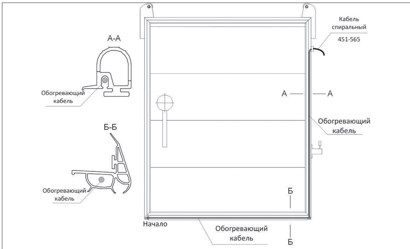
Схема установки нижнего контура обогрева полотна двери.
